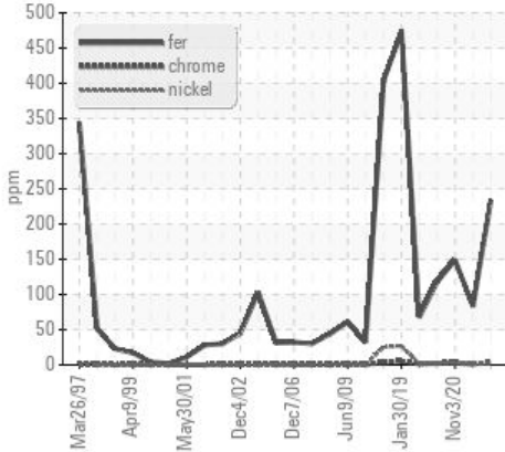
▲ Alliage ferreux
