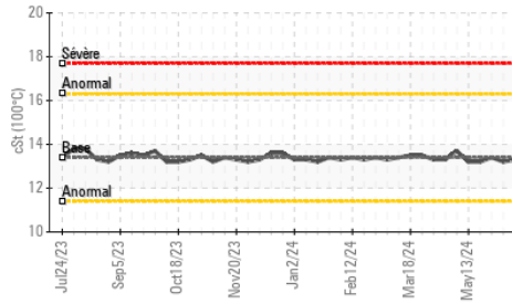
Viscosité 100°C
