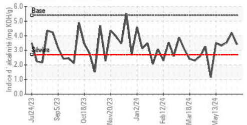
Indice d'alcalinité
