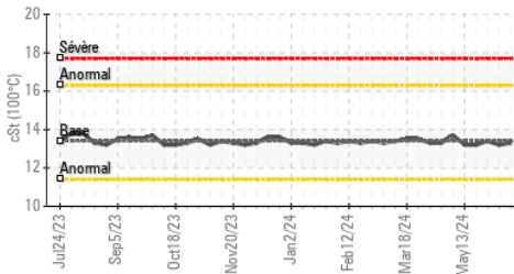
Viscosité 100°C
