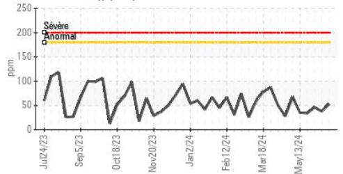
Indice d'alcalinité
